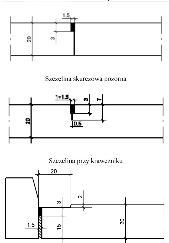
Rys. 1.1. Przykłady konstrukcji szczelin w podbudowie z betonu cementowego (wymiary w cm)
